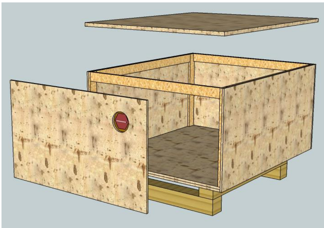
Abbildung 1: Plattenkiste AVL-Ausführung
