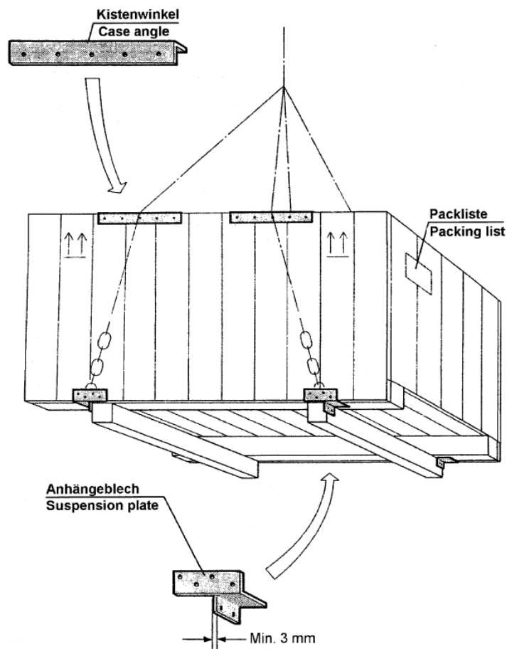
Abbildung 8: Darstellung ber die Anordnung der Schwergutbeschlge
