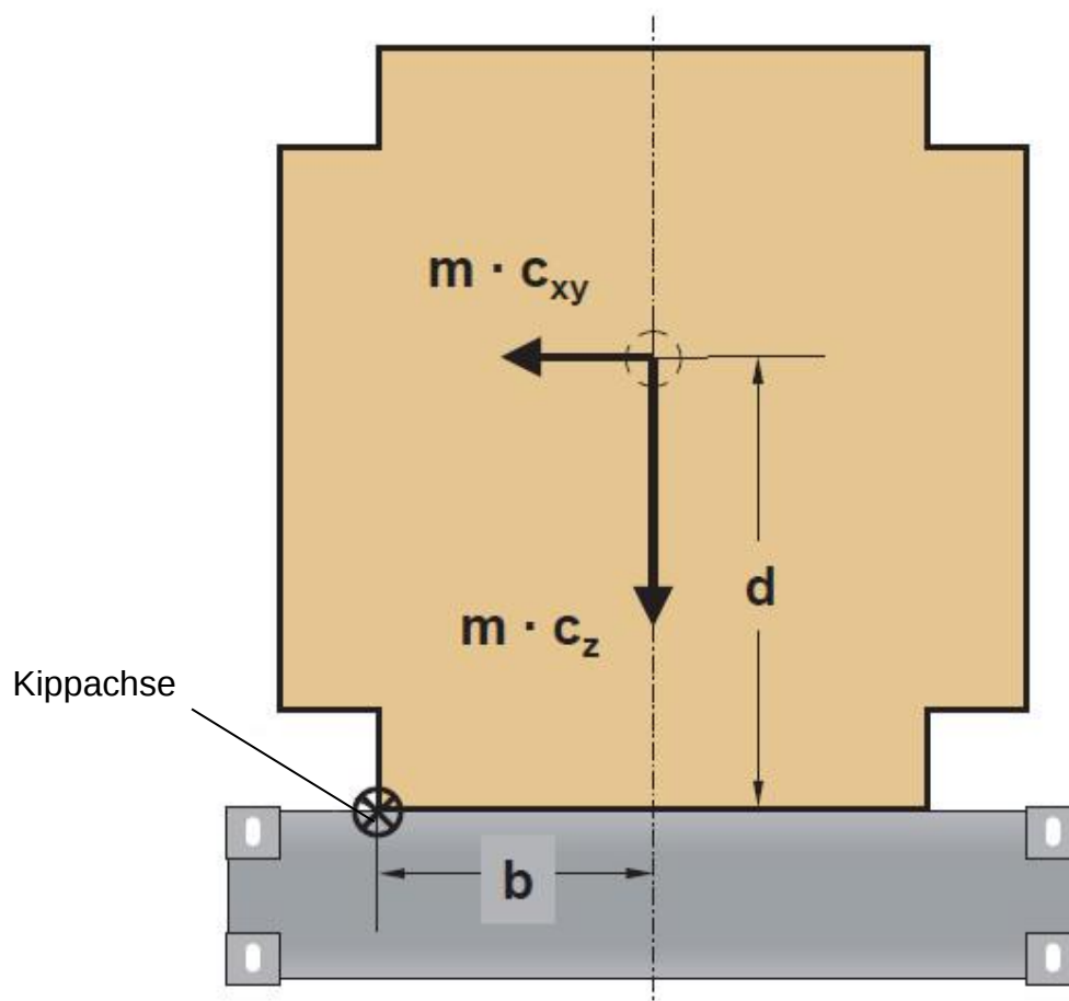
Abbildung 15: Kriterium für das Anbringen eines Kippindikators
